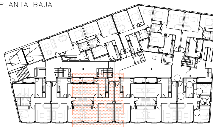
PLANTA BAJA
